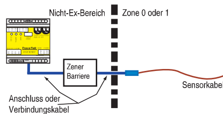
In Verbindung mit einer Ex geeigneten zugelassenen Zener-Barriere können TraceTek Sensorkabel in Ex- Zonen 0 und 1 verlegt werden.
